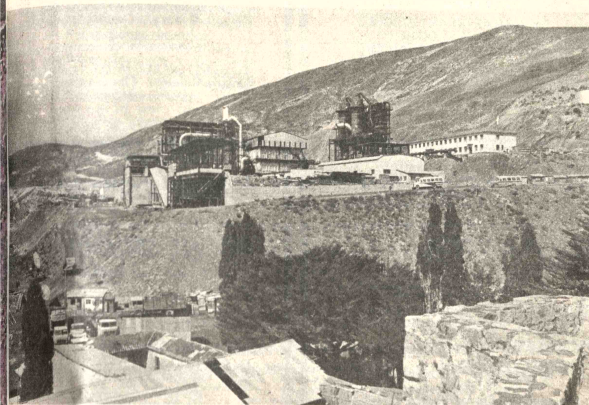
PLANTA DE VOLATILIZACIÓN.- La Planta de Volatilización de La Potosí, que preparará minerales de estaño de baja ley, para que puedan ser procesados en las fundiciones de Vinto, será inaugurada a fines de febrero. En su tipo, es la planta más grande del mundo, costó casi 70 millones de dólares, financiados por la URSS.
