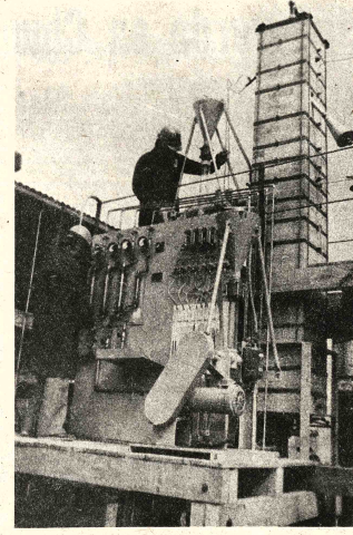
HORNO. En el Instituto de Investigaciones Minero Metalúrgicas, recientemente se ha instalado un horno de Lecho Fluidizado. La moderna maquinaria del IIMM hace posible ejecutar trabajos de investigación y crear nuevos procesos y sistemas mineros.
