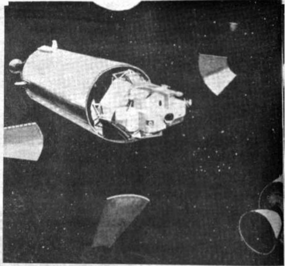
6.— Ahora, los astronautas voltean el vehículo espacial hasta que el extremo agudo apunta al Módulo Lunar. Mientras tanto, un mismo de muelles abre y desprende la cubierta de Módulo Lunar. Esta cubierta es llamada oficialmente Adaptador del Módulo Lunar de la Astronave.
