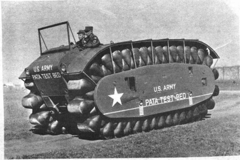
FLOTANDO SOBRE AIRE. Bolsas de aire hacen de orugas en este tanque para llevar tropas o carga, diseñado en los Estados Unidos. Su objeto es ser usado en el transporte sobre muchas clases de terreno, incluyendo arenales, pantanos, agua y caminos pavimentados o no.
