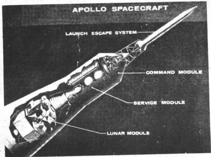
4.— Este esquema del vehículo Apolo muestra a los astronautas reclinados en sus asientos en el Módulo de forma de embudo. El Módulo Lunar (abajo) descansa dentro de una cubierta protectora. La torre de escape al lanzamiento (en la parte superior) se desprende cuando la astronave sale de la atmósfera.
