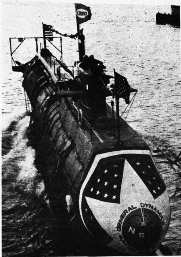
SUBMARINO NUCLEAR. — Este es el submarino NR-1, primer sumergible del mundo movido por energía nuclear que se dedica a las investigaciones, botado el 25 de enero pasado en Groton, Connecticut. Tiene 42 metros de largo y lleva siete tripulantes.
