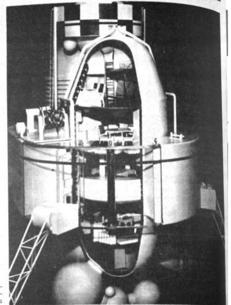
Vista de la parte donde se acomodará la tripulación de un aparato destinado a investigaciones profundas del mar. El dispositivo ha sido desarrollado por la Armada norteamericana. Los espacios del laboratorio están situados abajo y la tripulación en la parte superior. Las esferas almacenarán cámaras fotográficas y de televisión.
