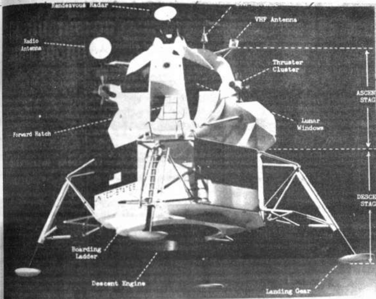
LEM.— La foto muestra algunas de las características del vehículo llamado Módulo Lunar que pesa 23 toneladas y mide 7 metros de altura. La mitad inferior, llamada sección para el descenso, se posará en la superficie lunar. Cuando los astronautas hayan completado su misión, esta sección se quedará en la luna, después de servir de plataforma de lanzamiento para la sección de ascenso.
