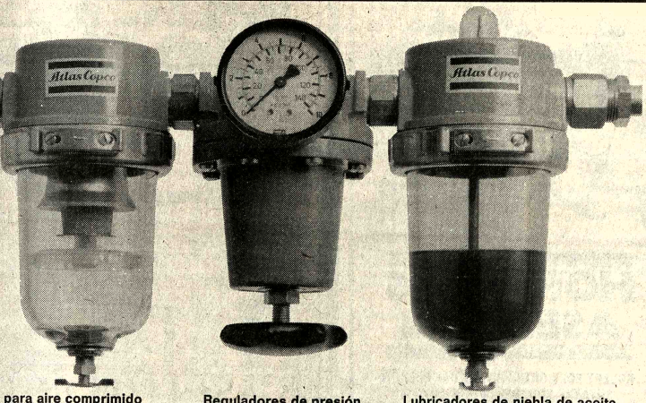
Filtros para aire comprimido Reguladores de presión Lubricadores de niebla de aceite
