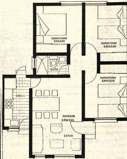
VIVIENDA TIPO "H" SUPERFICIE CONSTRUIDA = 68.50 M 2 -3 Dormitorios
