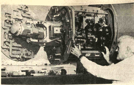
RADAR, CULVER CITY-CALIFORNIA (USICA). - El radar de proa del avión de combate Hornet F-18 es preparado para un vuelo de prueba en la fábrica Hughes Aircraft, aquí. El sistema de aire a aire, y de aire a tierra, está diseñado para proporcionar información de radar de toda altitud y de todo aspecto para permitir al piloto una variedad de órdenes contra blancos fijos y móviles. El F-18 se encuentra bajo desarrollo para la Fuerza Naval y el Cuerpo de Infantería de Marina de los EE.UU.
