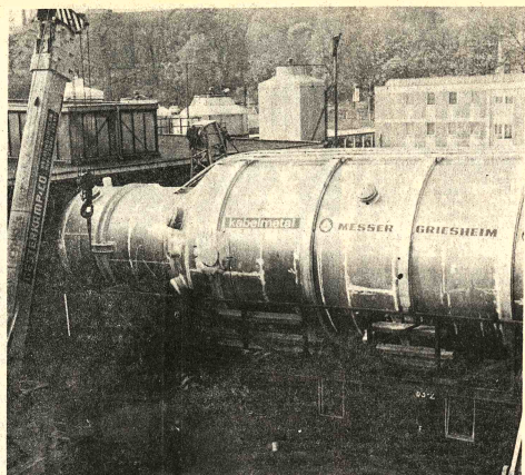
CONSTRUCCION. Oberhausen (did). Para la construcción de este depósito de casi 22 metros de longitud y 90 toneladas de peso, con un diámetro de 5,3 metros, es necesaria la máxima precisión y un perfecto know-how. Se trata de una columna de baja presión de aluminio con un volumen útil de 400 m 3 para presiones de trabajo de hasta 7 bares y temperaturas de 150 grados centígrados. (Foto did)
