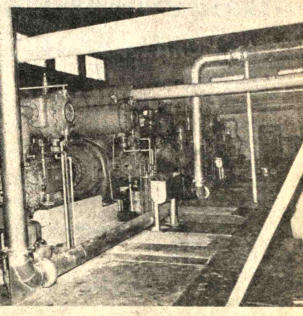
2. Tres compresoras inauguradas en la sección "Patillo" de Huanuni, cada unidad tiene una capacidad de 5.000 pies cúbicos de aire para provisión a interior mina. El costo total es de 7 millones 400 mil pesos bolivianos.
