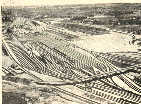
TORNABIAS. Hamburgo (INP/HIB) - Al sur de Hamburgo se está construyendo el mayor tornavía de Europa, la estación de maniobras Maschen. Este proyecto destinado al transporte de cargas norte-sur y sur-norte con 300 kilómetros de vías y 1.000 cambios, cuesta 80 millones de marcos a los Ferrocarriles Federales Alemanes (Foto INP).
