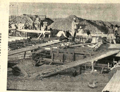
AMPLIACION. Se aceleran las obras civiles para la ampliación de la planta térmica de Aranjuez en los trabajos de encastrado.
