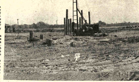
EN PALMASOLA: Sobre un campo alierito de 114 hectáreas de terreno plano empieza a levantarse paulatinamente la nueva refinería de Palmasola, a 10 kilómetros de Santa Cruz de la Sierra (FOTO PRESENCIA Santa Cruz).
