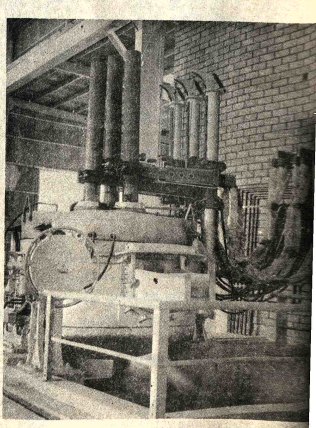
HORNO ELECTRICO TRIFASICO A ARCO VOLTAICO DIRECTO DE 1.500 KVA.
