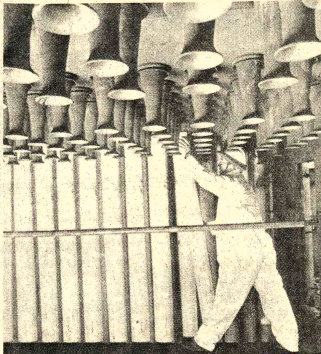
CONTAMINACIÓN: Gigantescos sacos filtran partículas de alumina en un neurótico sistema de control de aire contaminado, desarrollado por la Aluminum Company of America, en la planta de Wenatchee, Washington. El proceso de secamiento trata con el gas carbónico que se desprende de los hornos y que contienen hidrocarburos, polvo de carbón y fluoruros, descartando aire limpio. Este procedimiento elimina el uso de grandes cantidades de agua usadas en los sistemas húmedos (7-61).
