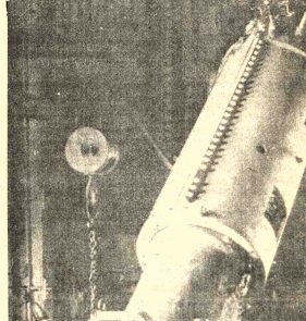
AJUSTE DE VALVULAS.- Preparación de una gigantesca válvula de vapor para uso de una planta nuclear para suministrar a prueba en la planta de Rockwell International, en Raleigh, Carolina del Norte. El dispositivo de control, de 27 toneladas, es el más grande de su tipo jamás construido. La Rockwell ha construido válvulas para las primeras plantas eléctricas comerciales con combustible nuclear en Shippington, Pensilvania, y el submarino Nautilus, así como para el primer buque mercante nuclear Savannah, U.S.S.
