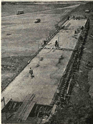
En un esfuerzo mancomunado el Comité Departamental de Desarrollo y Obras Públicas de Potosí y el Servicio Nacional de Caminos hicieron posible la construcción de este puente sobre el río Chaqui Mayu en la carretera Potosí - Sucre, el mismo que será puesto al servicio en fecha 15 de Noviembre de 1975.
