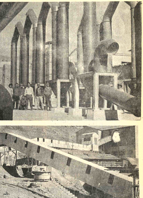
Esta es la única planta de preconcentración de mineral de Pallavi.
