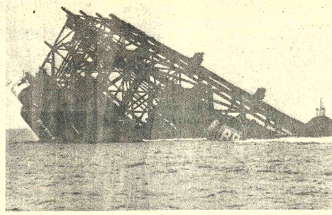
EN BUSCA DE PETROLEO.- Frente a la costa francesa.- 19 (AP). - La plataforma de la British Petroleum Company, Graythorpe, II, se inclina y se sumerge por colocarse luego en su posición correcta cuando llegue al lecho del Mar del Norte. La plataforma pesa 22.000 toneladas. Será usada para sacar petróleo del campo de Forties, uno de los más ricos del Mar del Norte. (Radiofoto AP).
