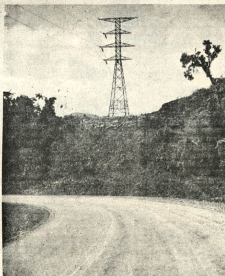
Imponente vista de una torre en la Línea de Transmisión Sta. Isabel - Corani.
