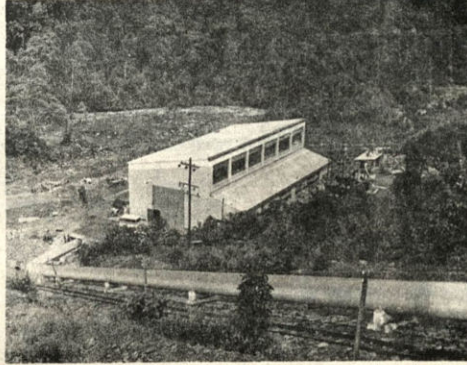
Vista lateral de la tubería de presión, casa de máquina y vista parcial de la sub-estación.
