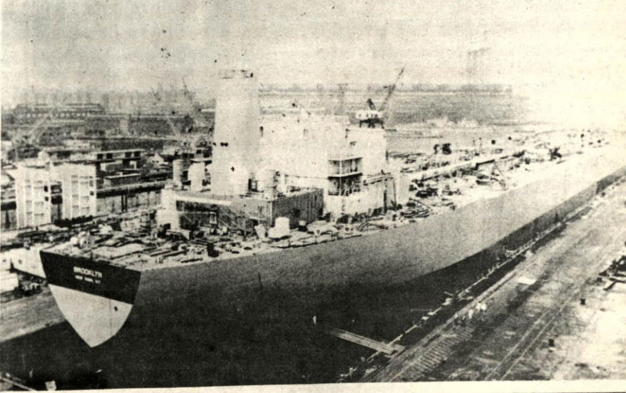
-Este es el T.T. Brooklyn, el mayor buque mercante construido hasta hoy en los Estados Unidos. El supertanque que pesa 225.000 toneladas, entrará en servicio a fines de este año. Fue construido en lo que era antes el astillero naval de Brooklyn, en la ciudad de Nueva York. El T.T. Brooklyn tiene una capacidad de carga de 1.500.000 barriles de petróleo. Mide 333 metros de largo.
