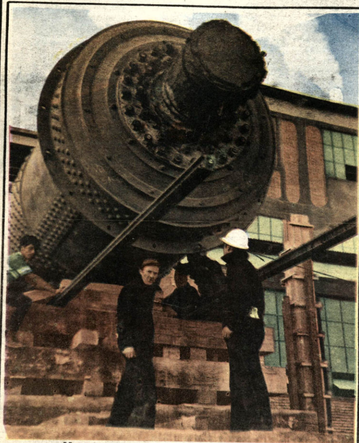
Montaje del gigante molino de cemento F.L. Smith accionado por el motor eléctrico más grande del país de 1.000 H.P.
