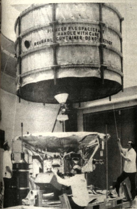
La nave espacial Pionero II en preparación para su embarque de una fábrica en California al Centro Espacial Kennedy, en Florida. Se espera que esta nave sea lanzada hacia Júpiter en abril de este año. El Pionero 10, el primero de los experimentos hacia grandes planetas del sistema solar, fue lanzado en marzo de 1972. Estos vehículos llevan instrumentos para recoger información y transmitirlos a la Tierra tanto de un tránsito como de las vecindades de los planetas por los que pasan.
