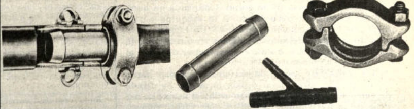
ABRAZADERAS Y MANGUITOS DE UNION DE MANGUERA
