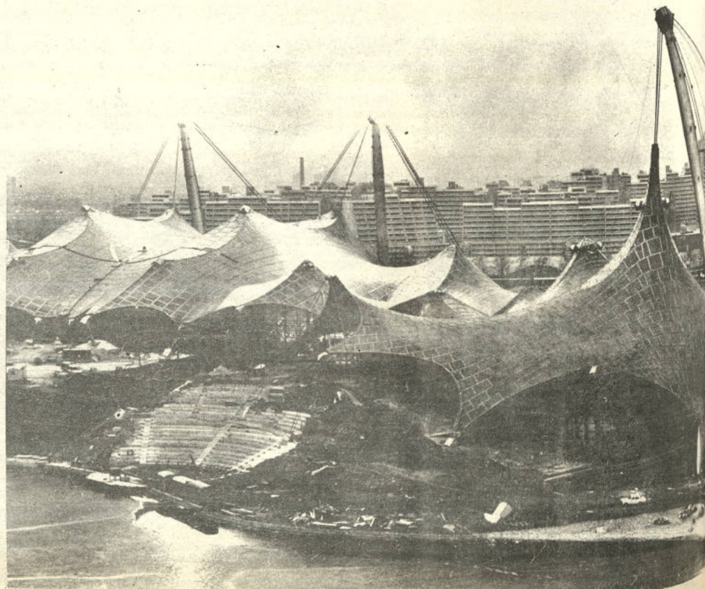
Palacio del Deporte para uso múltiple (izquierda) y estadio náutico (derecha). En el primer plano: el lago artificial y la tribuna al aire libre. En el fondo la Villa Olímpica.
