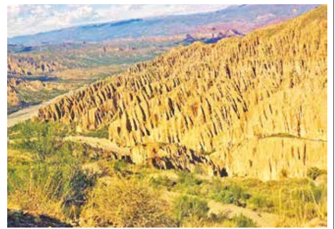
El Sillar atrae por sus formaciones geológicas.
