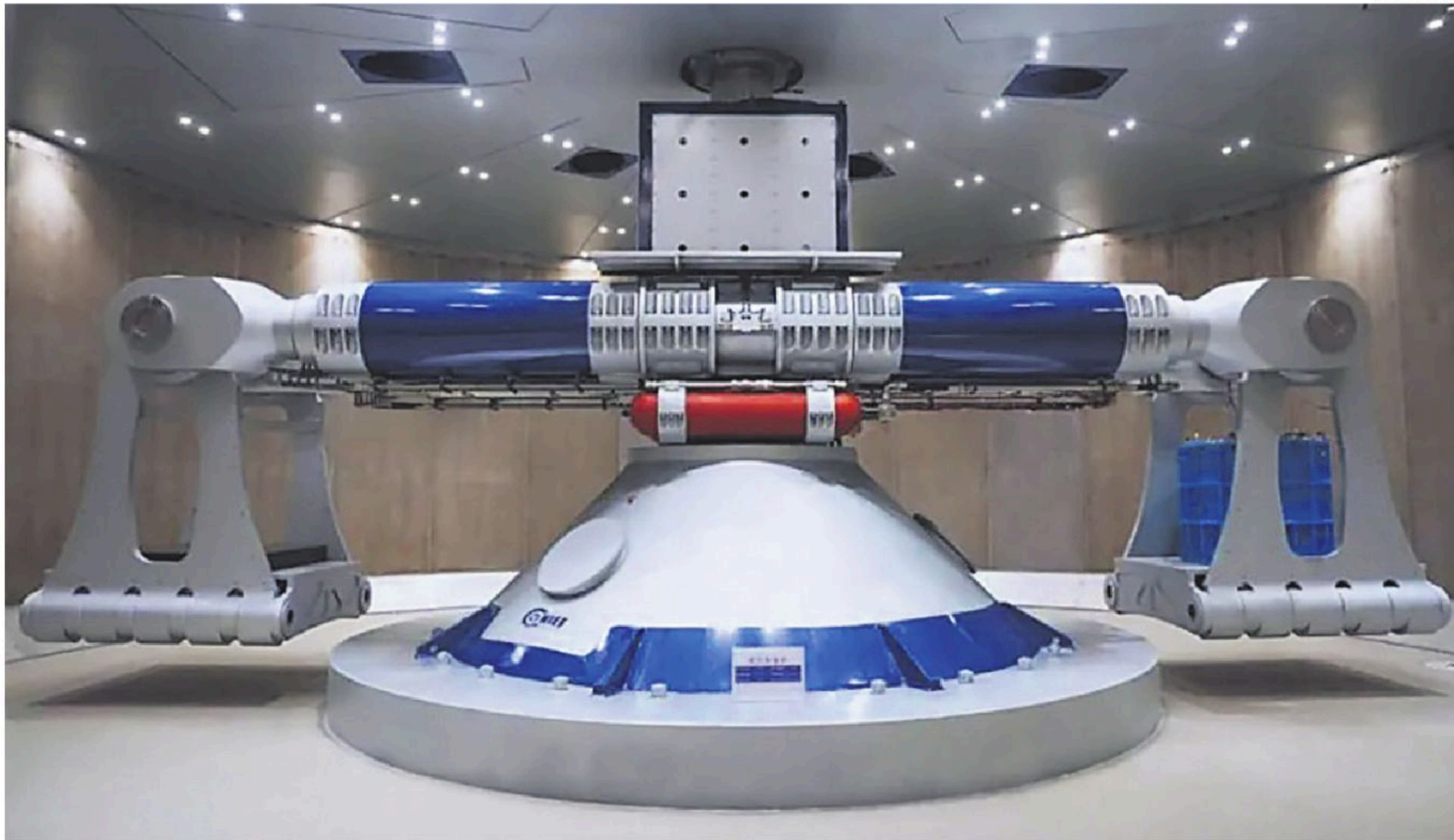
La centrifugadora de hipergravedad CHIEF1900 se encuentra instalada en la universidad de Zhejiang
