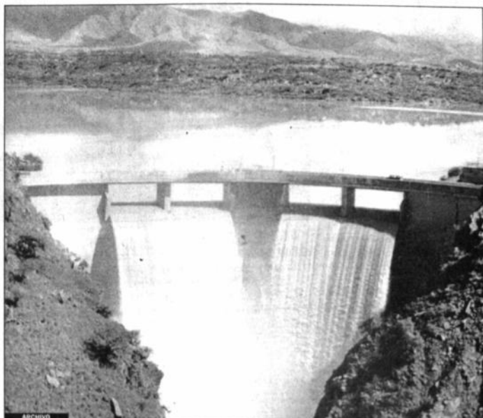
La represa de San Jacinto.
