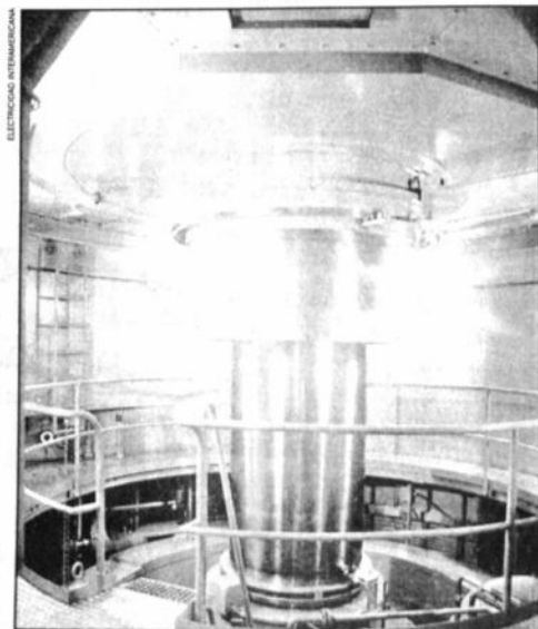
Eje de los generadores de la Central Colbún
