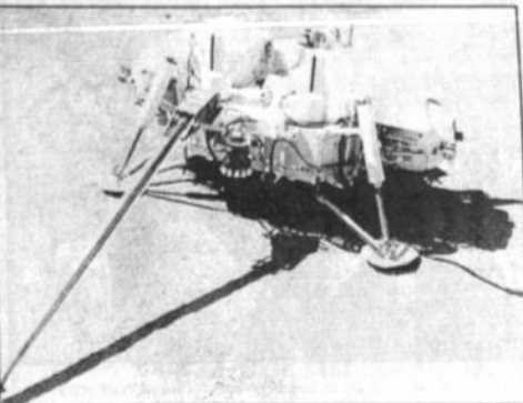
Una de las primeras naves Viking que llegó a Marte para realizar investigaciones científicas.
