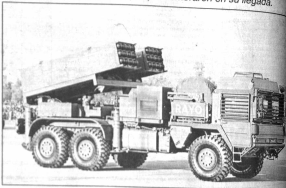
En el desfile militar realizado en Santiago de Chile se exhibió el moderno cohete Rayo, destinado a la exportación.
