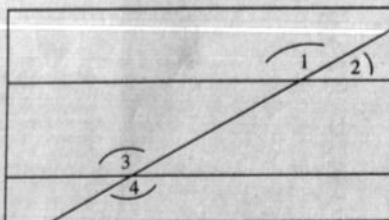
EL TEOREMA DE LOS ÁNGULOS INTERNOS Y EXTERNOS DETERMINADOS POR DOS RECTAS PARALELAS CORTADAS POR OTRA RECTA: ÁNGULOS 1-3 Y ÁNGULOS 2-4.
