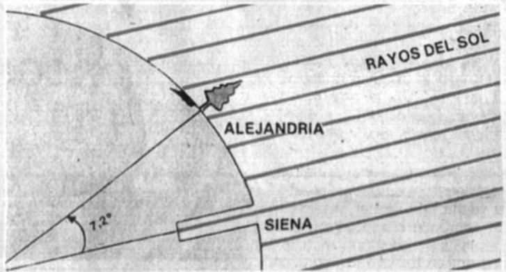
ERATOSTENES NOTO QUE CUANDO LA LUZ DEL SOL ENTRABA DIRECTAMENTE A UN POZO EN LA CIUDAD DE SIENA, EN ASUÁN (EGIPTO), UN OBELISCO EN ALEJANDRIA ARROJABA SOMBRA.
