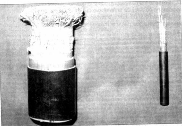
Cable de cobre (izq) y de fibra óptica (der). Ambos pueden llevar señales digitales, pero el último tiene mayor capacidad, ofrece más velocidad de transmisión y garantiza mejor fidelidad de la señal (foto: cortesía COTEL).
