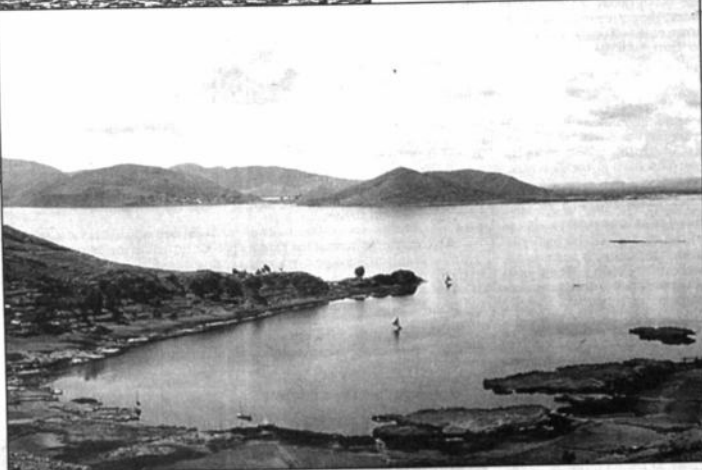
Suelos lacustres. Los lagos depositan en sus orillas materiales en suspensión.
