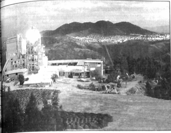
Con su quinta ampliación, la Fábrica Nacional de Cemento (FANCESA) será la industria líder en el país. Sus directivos y los sucesores están resueltos a llevar adelante, contra viento y marea, un proyecto largamente postergado
