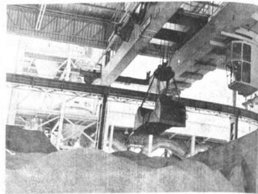
Una grúa puente traslada la piedra caliza salido de la chancadora hasta los hangares de almacenamiento y ejecuta una mezcla preliminar de la materia prima que será transformada en cemento.
