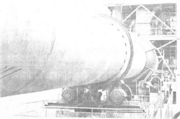
El horno cilíndrico que se mantiene en constante movimiento de rotación, conserva en su interior una temperatura que va de los 800 a los 1450 grados centígrados. Personal especializado realiza el trabajo de vigilancia que se desarrolla durante las 24 horas del día.
