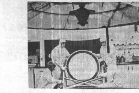
OJO COPERNICO.-Estas es el espejo telefónico primario de 82 centímetros, parte del experimento ultravioleta de la Universidad de Princeton, que se encontraba a bordo del Observatorio Astronómico en órbita (sigla en inglés OAO-3), cometido ahora a bordo en el Centro Espacial de Goddard, en Maryland, antes de su embarque a Florida para su lanzamiento.
