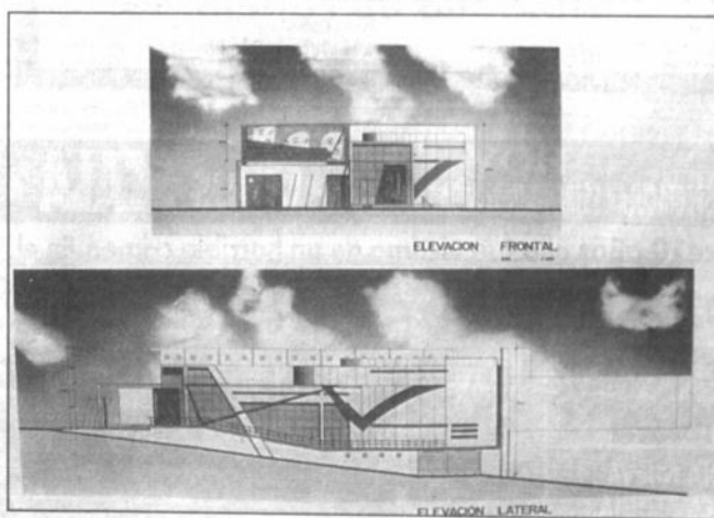
Dos vistas de lo que será la nueva Cinemateca Boliviana, según la concepción de los arquitectos Cecilia Sholz y Juan Carlos Aranibar, ganadores del concurso nacional de proyectos.
