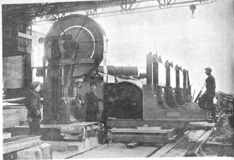
Aserradero de sierra sin fin "Stenner", tipo VQ72/CH57.
