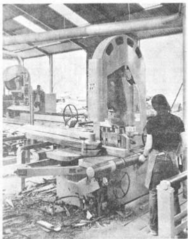
Sierra secundaria sin fin "Stenner", tipo VHL 48
