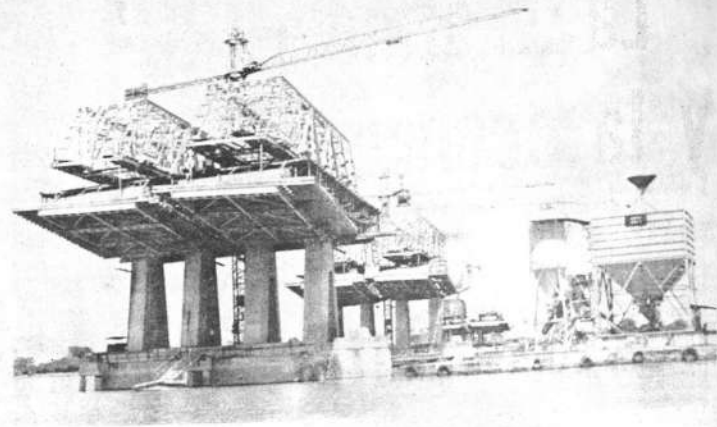
Puente sobre el río Guayas, Ecuador.
