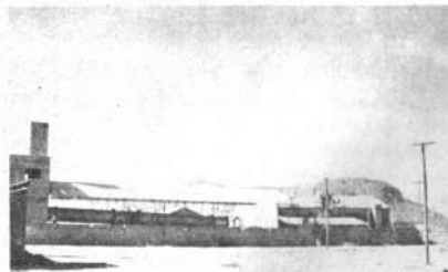
PLANTA CALCINACION MAGNESITA
