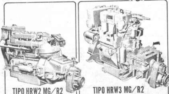
TIPO HRW2 MG/R2 29,5 HP 2200 RPM.
