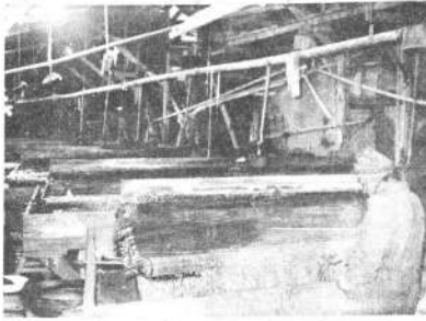
INGENIO DE MOROCOCALA.- El ingenio de Morococala trabaja permanentemente y en las diferentes secciones el mineral es tratado. En la fotografía, un obrero controla el funcionamiento de las mesas de concentración.
