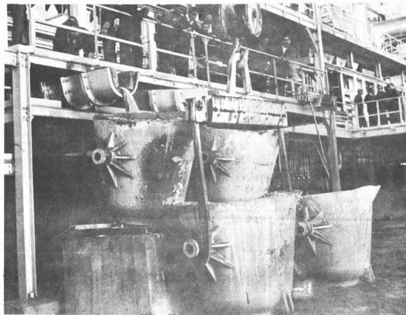
PROCESO.- En la Empresa Nacional de Fundiciones de Yinto se utiliza sistemas tecnológicos avanzados. En la fotografía se puede observar los hornos reverberos y los crisoles.
