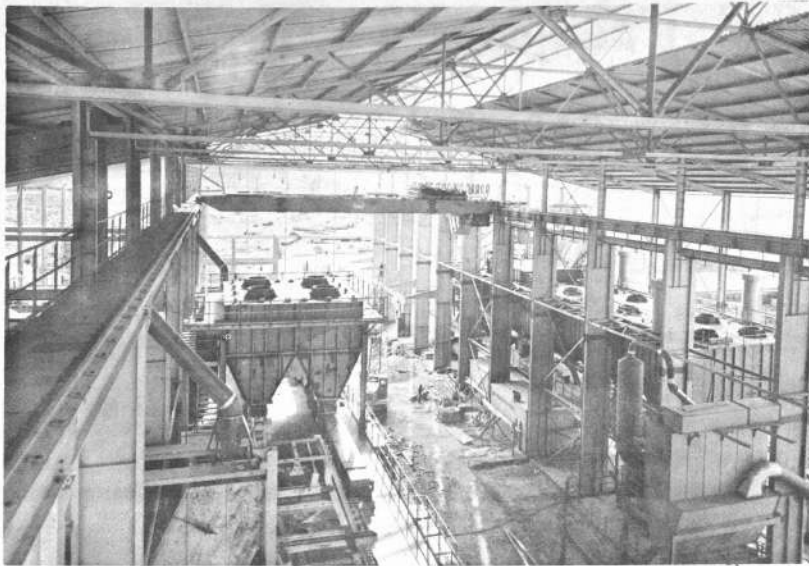
La construcción de las instalaciones de la Empresa Nacional de Fundiciones demandó el concurso de personal técnico especializado que bajo la dirección de ingenieros alemanes trabajaron intensamente. En la fotografía se observa el interior de la Nave de Fundición. Los hornos actualmente funcionan las 24 horas del día fundiendo estaño metálico.
