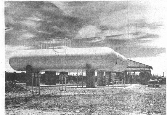
PLANTA ALMACENADORA DE GAS. Estos tres tanques de almacenamiento para gas licuado han sido instalados en El Alto de La Paz, y permitirán tener una reserva de 90 mil kilos. Adelante, se advierten las tuberías de transferencia destinadas a dos tanques más que serán instalados el presente año. Al fondo, se ve el tinglado donde se engrasará y guardará el producto envasado. La planta fue inaugurada ayer oficialmente.
