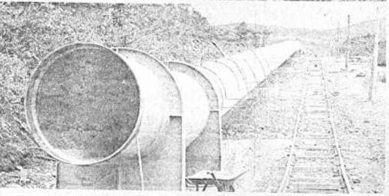
El trabajo en ensamble consta de varios pasos, arriba: desde este lugar comenzará el túnel. Al centro parte de la tubería instalada. Abajo, sitio de los trabajos actuales.
