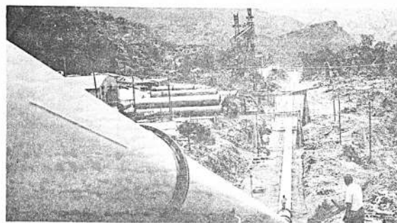
Un tramo de la tubería de presión, mostrando la inclinación.
