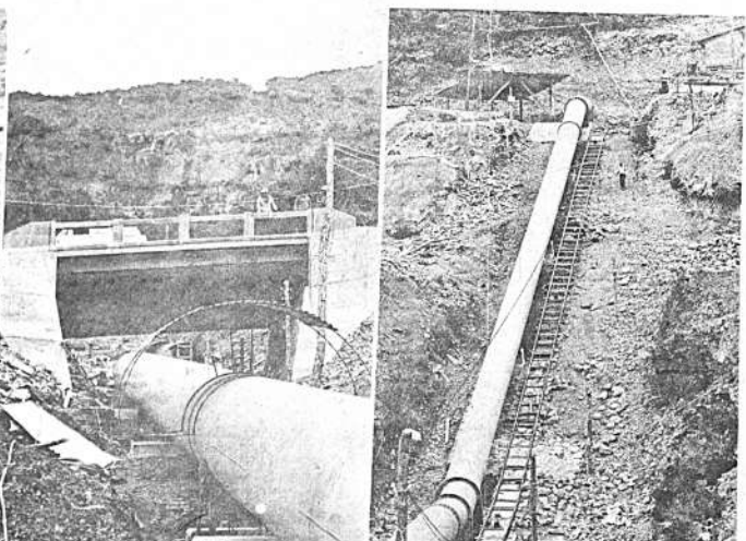
Distintas etapas de la colocación de la tubería, a la derecha se puede observar la línea de transporte.
