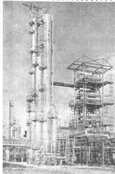
Planta Petroquímica y Refinería de Viena.
