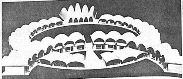
ESCUELA NORMAL "ENRIQUE FINOT". El Departamento de Arquitectura del Consejo Nacional de Edificaciones Escolares ha hecho la maqueta del moderno edificio de la Escuela Normal Enrique Finot de la ciudad de Santa Cruz. Arriba, en la fotografía la maqueta del edificio que se está construyendo por los arquitectos Juan Luis Zuhiga y Rodolfo Albarito.
