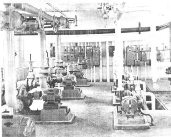
Esta serie de válvulas y el sistema de tuberías muestran un aspecto imponente en la serie de máquinas de la planta generadora de ENDE en Santa Cruz.
