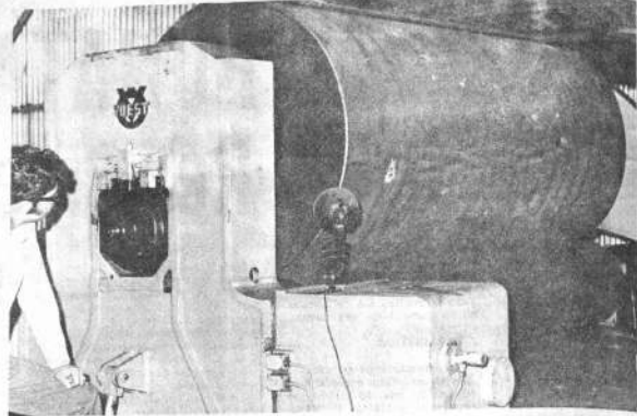
Una de las chapas metálicas de tres toneladas y medio luego de haber sido sometida a la máquina dobladora adquiere la forma requerida
