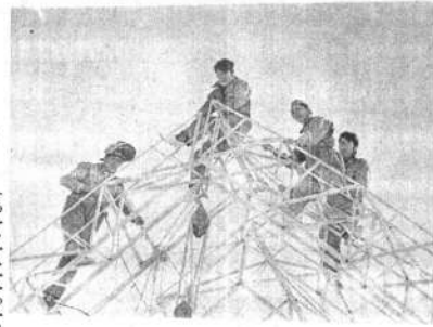
Trabajadores especializados de "Camena", colocan la estructura metálica para el techo de la nueva Catedral de Oruro. La estructura mide 26 metros de altura desde el nivel del edificio en construcción.
