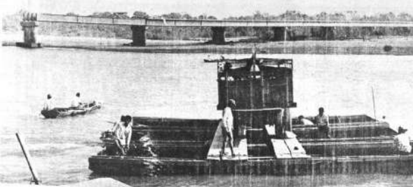
Una vista panorámica del puente sobre el río Yapacaní, cuyos trabajos quedaron postergados desde hace dos años. Se puede observar que la izquierda el puente está incompleto. El diseño final permitirá que esta obra se reinicie con el financiamiento de USAD y Bolivia.
