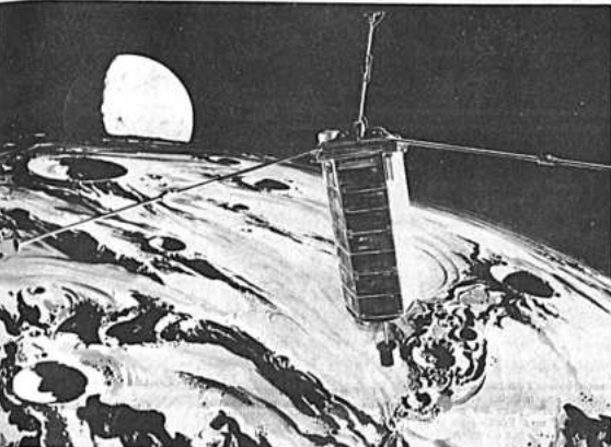
Este dibujo muestra el pequeño satélite que se pondrá en órbita alrededor de la Luna, el cual irá a bordo de la nave espacial Apolo 15. Será puesto en órbita por medio de un mecanismo de resorte, que será accionado poco antes de que se encienda el sistema de propulsión del módulo de servicio para el viaje de regreso a la tierra. Los sensores instalados en dicho satélite recogerán y transmitirán a la tierra datos sobre los campos magnéticos de la Luna, y proporcionarán un blanco al radar instalado en la tierra para estudiar el campo gravitacional de la Luna con la mayor precisión lograda hasta ahora. Tales datos unidos a los que enviaron los instrumentos dejados en la Luna por los tripulantes del Apolo 15, darán a los geofísicos una mayor comprensión de cómo sea posiblemente el interior de la Luna. El satélite estará dando vueltas alrededor de la Luna por un año.
