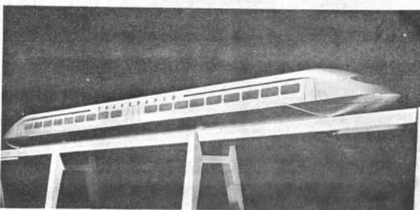
EL TREN DEL FUTURO: Un modelo del tren proyectado por Krauss-Maffei SA. de Munich, que alcanzará la velocidad de 457 Km/Hora.
