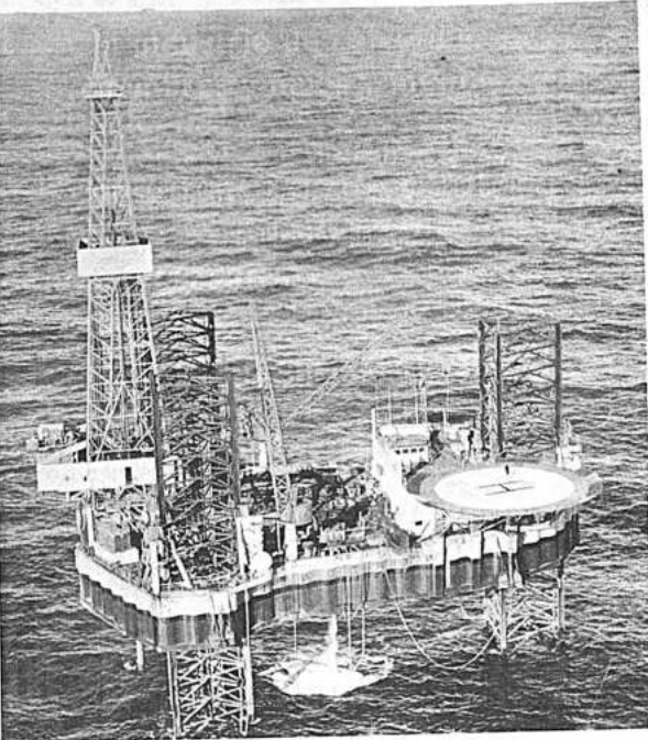
Plataforma "Nettuno I" para la búsqueda petrolífera de hidrocarburos en el Mar del Norte.
