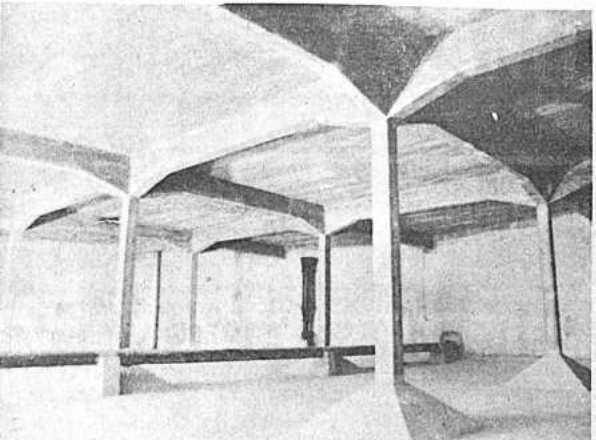
Como una inmensa catedral destaca el interior de uno de los tres estanques de almacenamiento de dos millones de litros cada uno con que cuenta el sistema.
