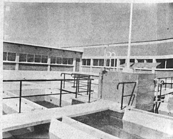
Planta de tratamiento de EL ROLLO. En primer plano los filtros y a continuación el decantador y el fondo la casa de aireación. En el lado izquierdo se destaca los edificios de explotación y grupos electrogénos. La capacidad de tratamiento de la planta, de 450 M3 por hora que permitirá proveer de agua a la población.
