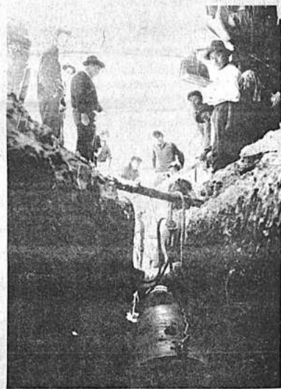
El encargado de obras Constantino Quiñones ejecuta el tendido de tubería de 350 mm. en la calle Junín, una de las más congestionadas de la ciudad.
