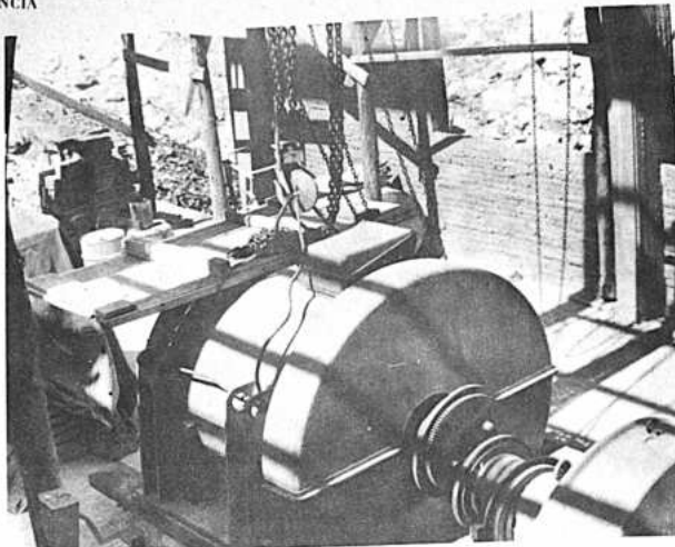
Una vista de las instalaciones de la planta hidroeléctrica de "Ruffo".
