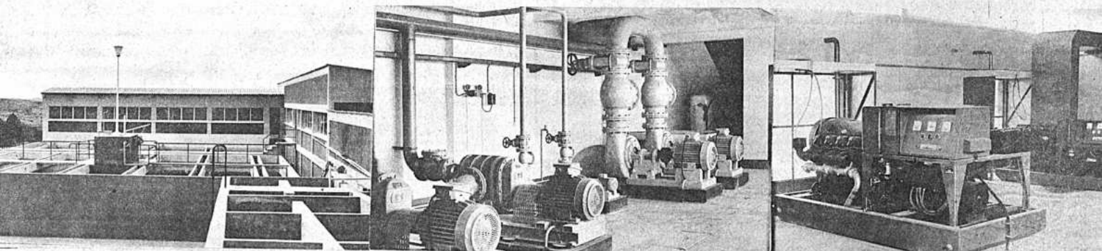
Vista Parcial de la Planta de Tratamiento de Agua destacan- dose el sedimentador y al fondo el edificio de la galería de filtros que permite la purificación de 480 metros cúbicos por hora.
