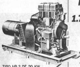
TIPO HR-3 DE 20 KW.
